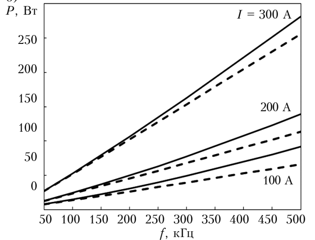
Рис. 5. Залежність втрат в перетворювачі від частоти з урахуванням втрат на індуктивності та без їх урахування (штрихові лінії) за різних значень вихідного струму I та напруги:
