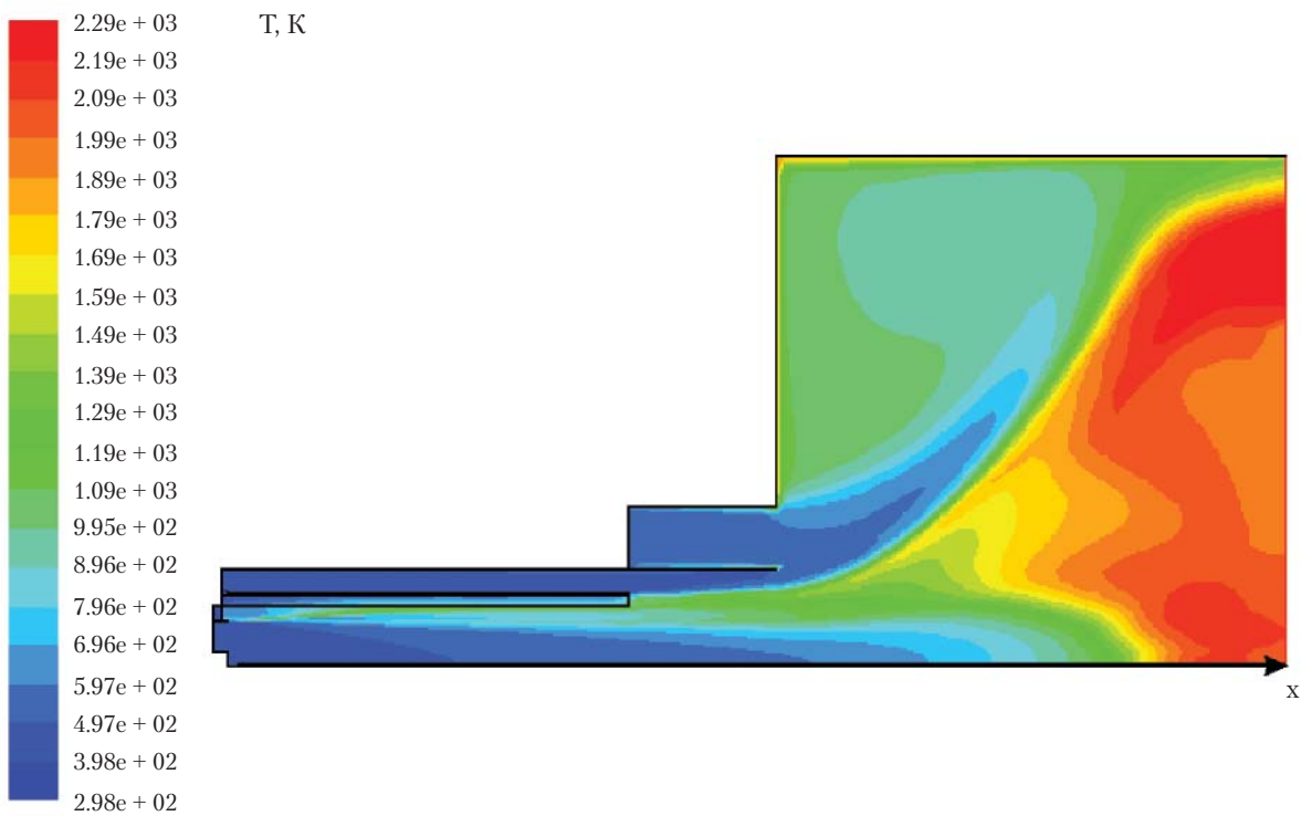
Рис. 3. Поле температур газової фази потоку в перерізі X–Y-пальника
