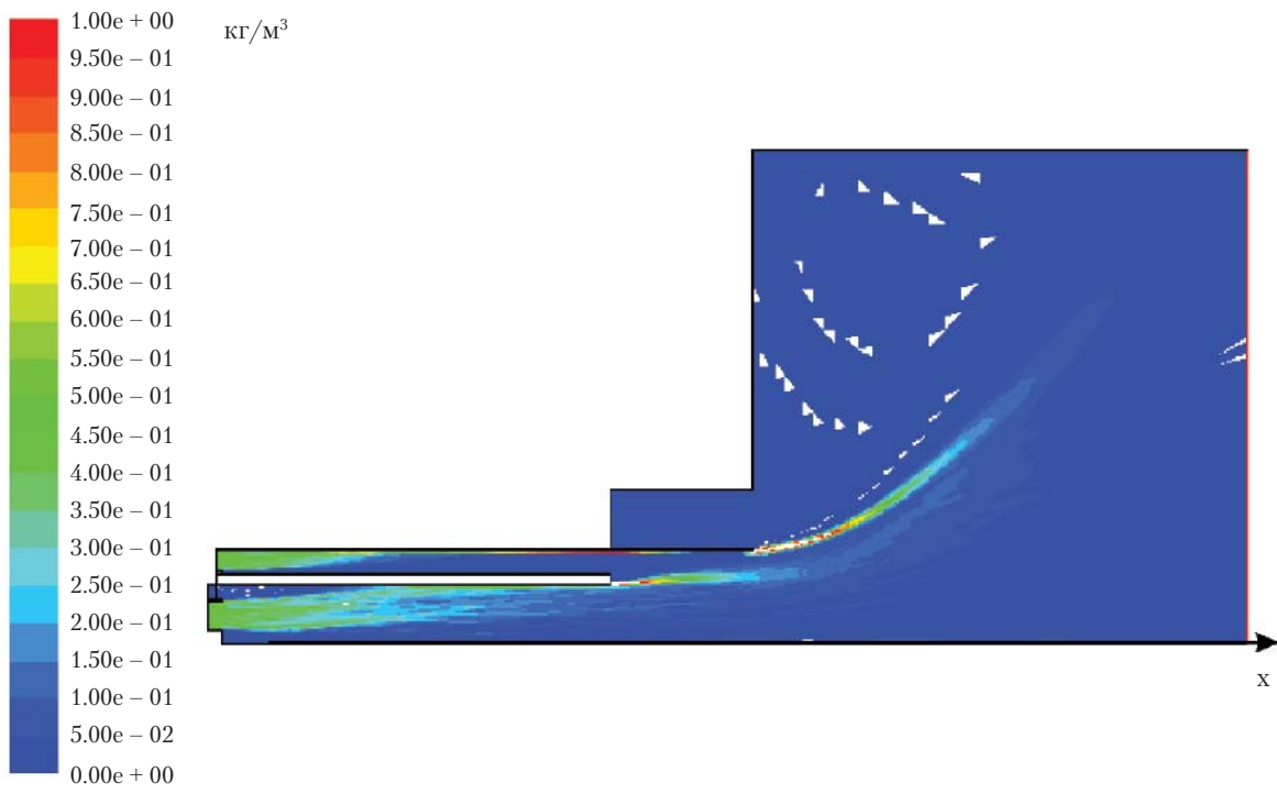
Рис. 4. Поле концентрацій вугільних часточок в завихрених потоках аеросумішей I і II
