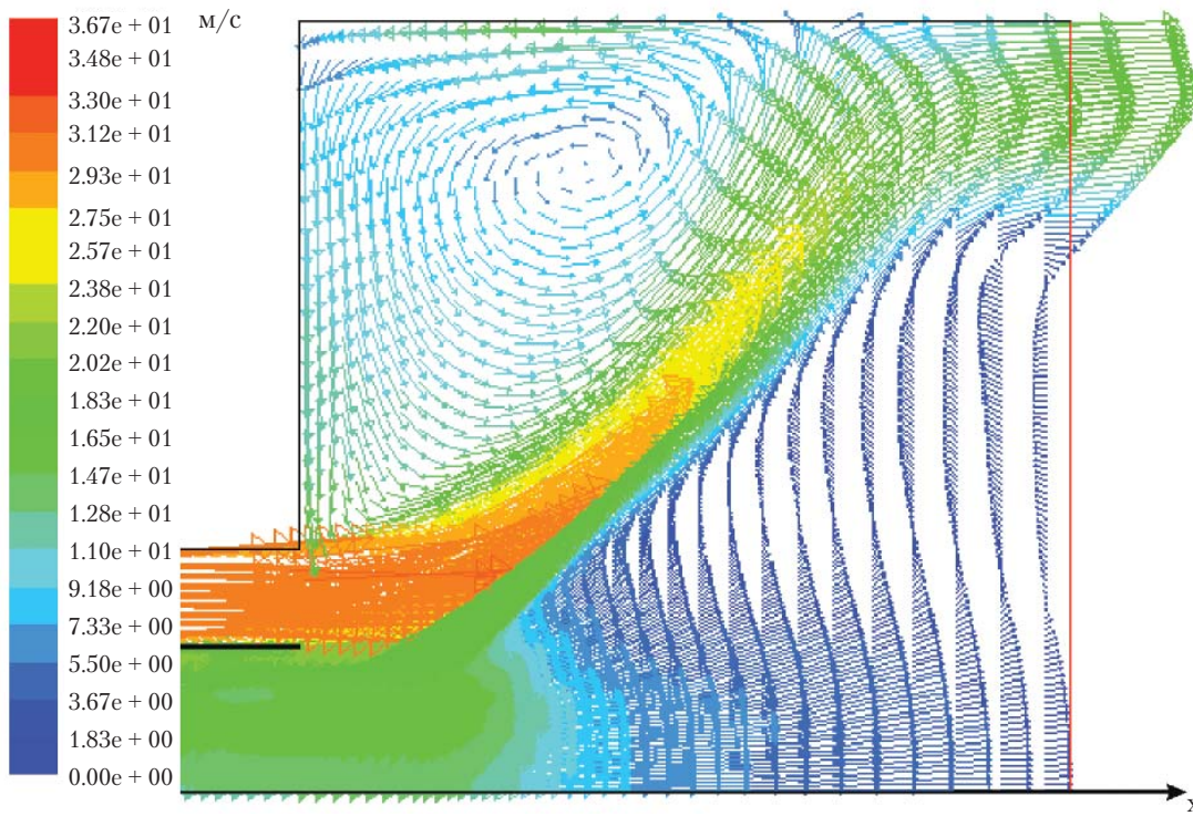
Рис. 2. Вектори швидкості вихідного потоку з пальника і зворотних течій топкових газів в площині X–Y
