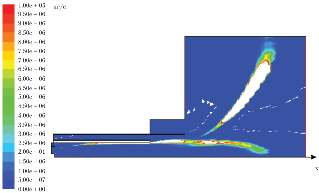
Рис. 5. Зони виходу летких у камері системи ТХІІ і в топковому просторі
