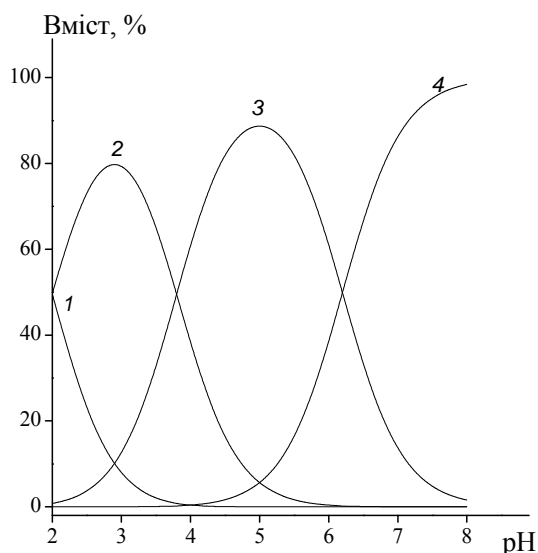
Рис. 2. Діаграма розподілу частинок АМФ в розчині в залежності від рН: повністю протонувана форма \text{H}_3\text{L}^+ (1), цвітер-іон \text{H}_2\text{L}^{\pm} (2), аніон \text{HL}^- (3) і діаніон \text{L}^{2-} (4).
