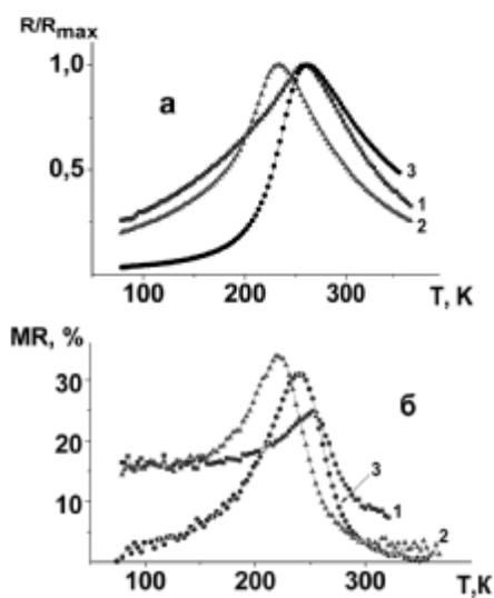
Рис. 2. Зависимость нормированного сопротивления ( a ) и магнитосопротивления ( б ) от температуры для пленки \text{La}_{0.775}\text{Sr}_{0.225}\text{MnO}_3 , напыленной на подложки \text{LaAlO}_3 (1); \text{Ba}_{0.996}\text{Y}_{0.004}\text{TiO}_3 (2); \text{BaTi}_{0.85}\text{Sn}_{0.15}\text{O}_3 (3).
