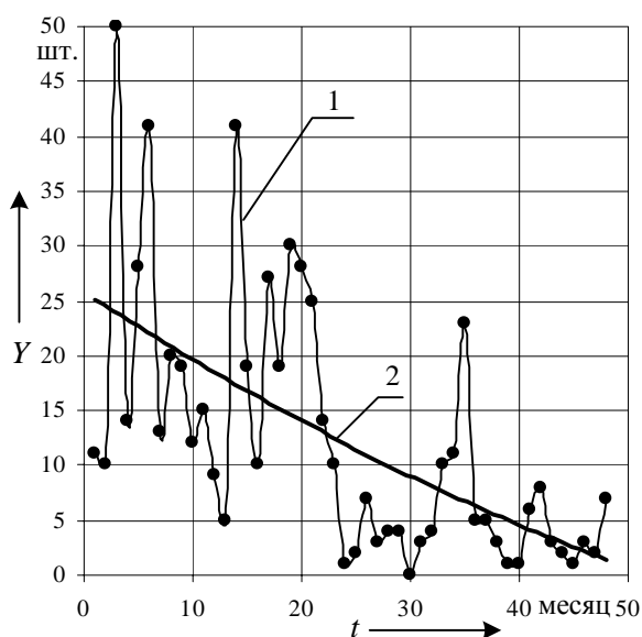
Рис. 4. График помесечного спроса и кривая роста на "общепромышленные" МПТ
