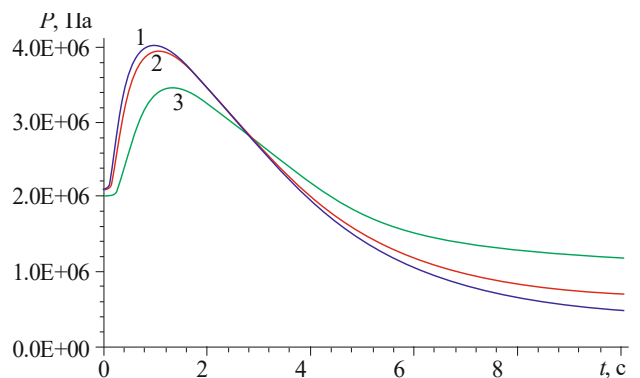
Рисунок 7. Изменение во времени давления газа на различном удалении \Delta x от контура выработки: 1 – 0.5 м; 2 – 1 м; 3 – 2 м
