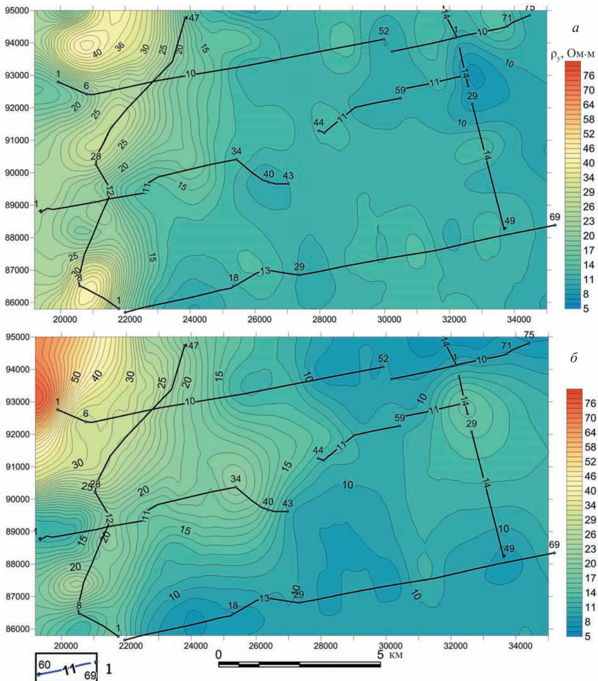
Рис. 6. Карты значений уявного опоры для разностей AB = 20 м у 2008 (а) та 2012 рр. (б): 1 – профіль ВЕЗ та його номер, номери кінцевих точок ВЕЗ
