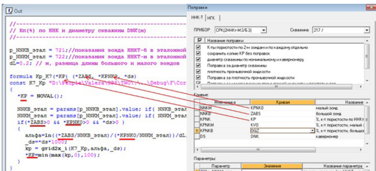
Рис. 5. Замена имён кривых, записанных в формуле, на имена, указанные пользователем Fig. 5. Replace the names of the curves recorded in the formula to the names specified by the user
