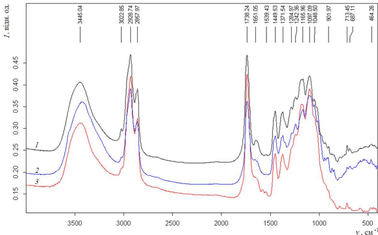
Рис. 3. ІЧ-спектри епоксидних композитів: 1 – вихідного епоксидного полімеру, 2 – з додаванням графіту, 3 – з додаванням полісилоксанових частинок і графіту
