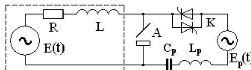
Рис. 2. Схема источника питания переменного тока со стабилизатором в виде LC-контур
