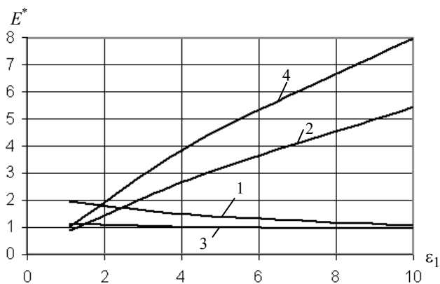
Рис. 6. Зависимость относительной максимальной напряженности электрического поля соответственно на криволинейных границах электрода (1) и раздела диэлектрических сред (2) от \varepsilon_1 при отношении r/d = 0,1 ; 3,4 - при r/d = 1
