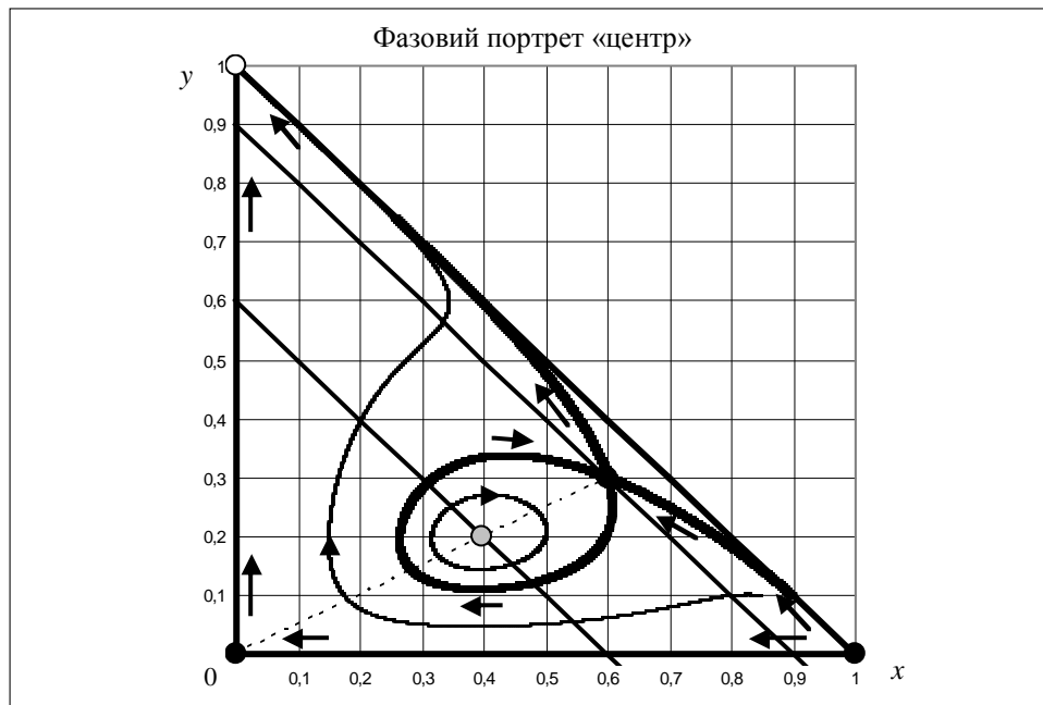
Рис. 4. Сценарій «компроміс»
