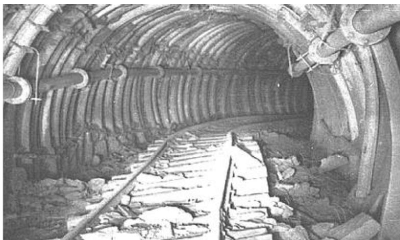
Рис. 11. Обходная выработка западного полевого квершлага гор. 1012 м шахты им. Бажанова ГП «Макеевуголь»
