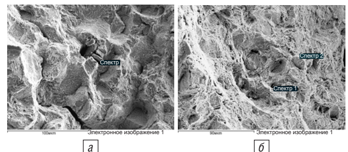
Рис. 2. Типичные поверхности разрушения разрывных образцов: \psi < 25 % (а); \psi > 25 % (б)
