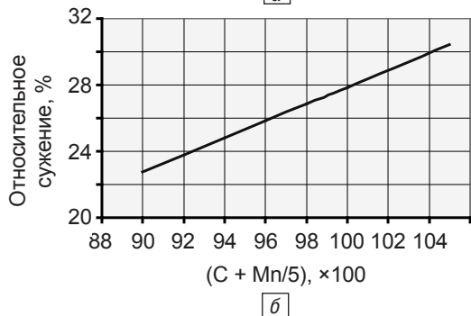
Рис. 6. Изменение относительного сужения от факторов химического состава: содержания кислорода (а); суммы содержания углерода и содержания марганца, деленного на 5 (б)
