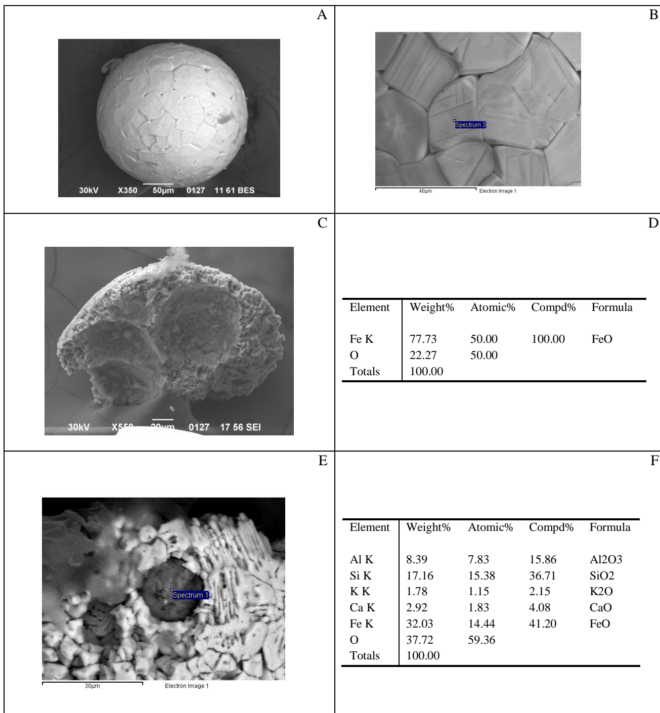
Рис. 8. Болидний шарик с диаметром 0,3 мм – (A); его поверхность– (B); округлые полости внутри разбитого шарика– (C); химический состав его вещества по РСМА, соответствующий вюстититу с вrostками металлического железа – (D); включения с диаметром 10-20 µм– (E); химический состав включения, соответствующий фаялит-герцинитовому парагенезису– (F).
