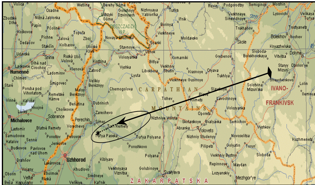
Рис. 2. Карта-схема и параметры траектории полета болида «Турья Реметы» [11].
