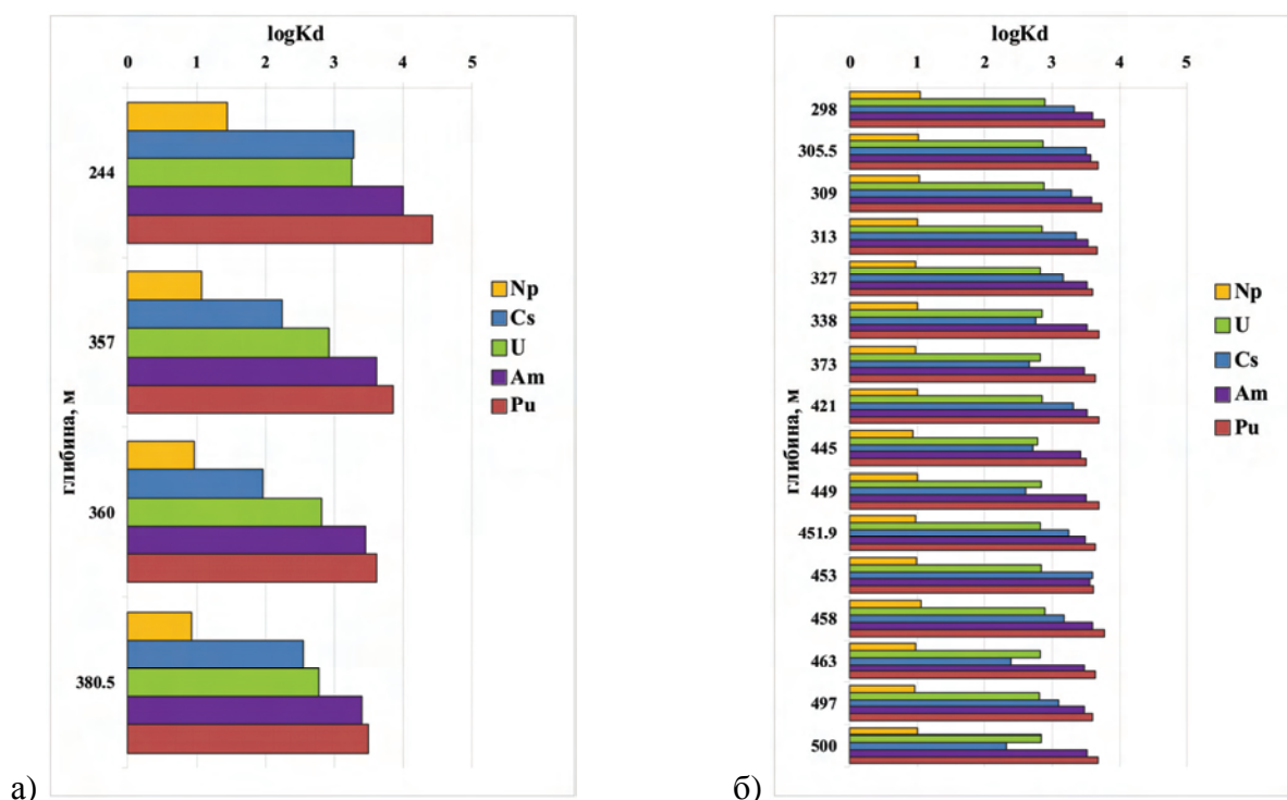
Рис. 2. Коефіцієнти розподілу U, Pu, Np, Am та Cs в гранітах та гранітоїдах при рН=7.5: а) – свердловина 50; б) – свердловина 35
