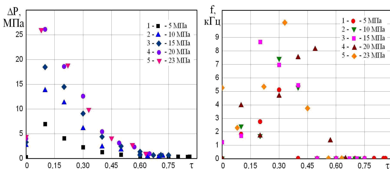
Рисунок 2 – Экспериментальные данные изменения размаха \Delta P и частоты f автоколебаний от параметра кавитации \tau для ГК-2,5 с \beta=35^\circ , l_{кр}=6,0 мм
