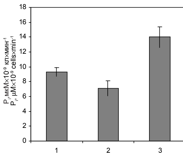
Рис. 2. Влияние замораживания-отогрева и отмывки на состояние \text{Ca}^{2+} -АТФазы эритроцитов: 1 – нативные клетки; 2 – клетки после замораживания-отогрева; 3 – клетки после завершения многоэтапной отмывки глицерола.
