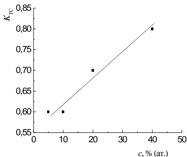
Рис. 1. Залежність коефіцієнта термостабільності алмазного порошку, синтезованого в системі Mg–Zn–B–C, від концентрації бору у вихідній шихті
