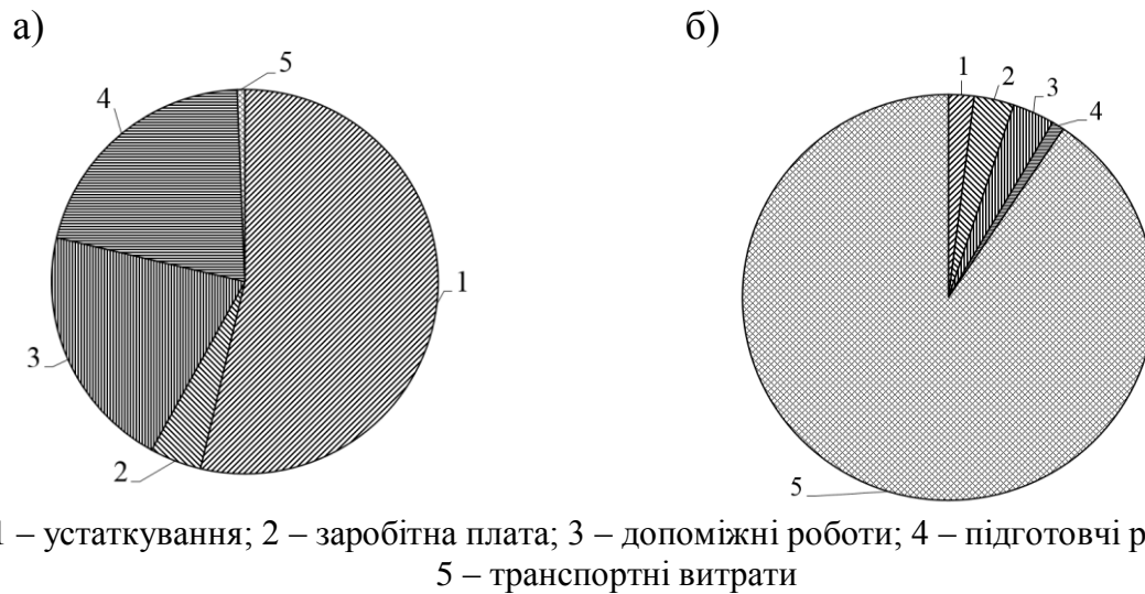
Рисунок 2 – Складові витрат, пов'язаних з видобутком урану двома порівняльними способами: а – підземний спосіб видобутку; б – комбінований спосіб видобутку (підземна розробка з використанням геотехнології)
