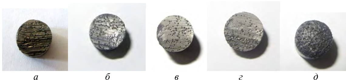
Рис. 2. Загальний вигляд експериментальних породоруйнівних елементів (вид згори), оснащених алмазами зернистістю : а – 400/315 \text{ мкм} не гранульованими АС 300Т (№ 1); б – 400/315 \text{ мкм} механічно вкритими гідридом титану АС 300Т (№ 2); в – 400/315 \text{ мкм} , обробленими іоноплазмовим покриттям титаном АС 160Т (№ 3); г – 400/315 \text{ мкм} механічно покритими хромом АС 300Т; д – 600/530 \text{ мкм}
