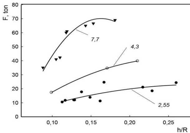
Рис. 2. Зависимости усилия сжатия диска R = 10,5\text{ мм} от его относительной толщины для различных материалов при заданном давлении в центре диска [4;5]
