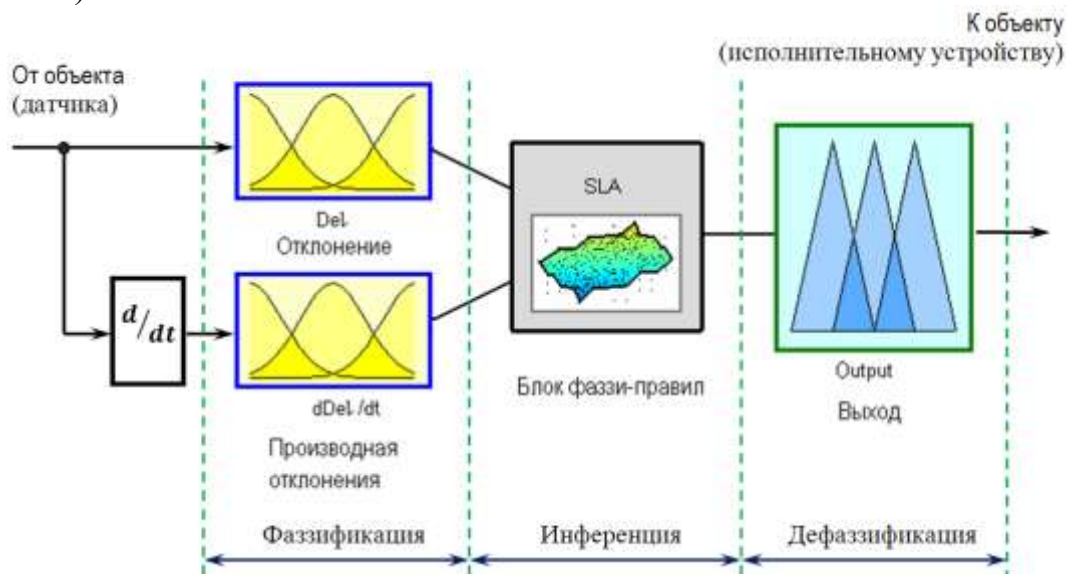
Рисунок 1 – Структурная схема фаззи-блока разрабатываемого контроллера
