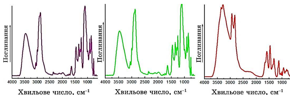
Рис. 2. ІЧ-спектри \text{LiClO}_4 (а), ДЕГ (б) і ПЕПА (в). 2
