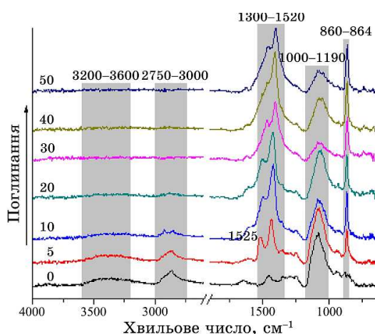
Рис. 3. ІЧ-спектри (в плівках) зразків композиційного матеріалу з різним вмістом солі перхлорату літію (м.ч.). 5
