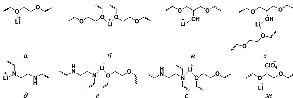
Рис. 4. Схеми можливих комплексів в системі ДЕГ-1/ПЕПА/ \text{LiClO}_4 . 6
