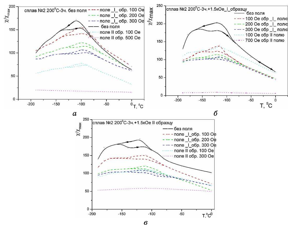
Рис. 2. Температурные зависимости низкополевой магнитной восприимчивости сплава Cu–Al–Mn после отжига при 200°C в течение 3 час.: а) без поля; б) в перпендикулярном поле; в) в параллельном поле; стрелками показаны нагрев–охлаждение. 2
