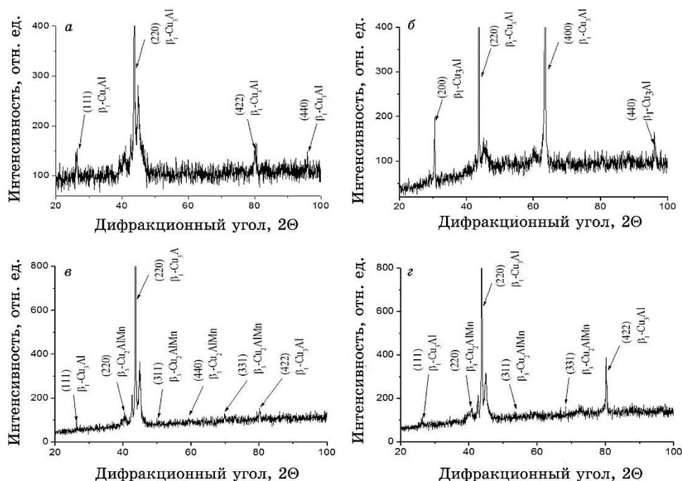
Рис. 1. Дифрактограммы образцов сплава CuAlMn, полученные в монохромном излучении Cu-анода: а ) после закалки; б ) после отжига без магнитного поля; в ) после отжига в перпендикулярном главной оси образца магнитном поле; г ) после отжига в параллельном главной оси образца магнитном поле. 1
