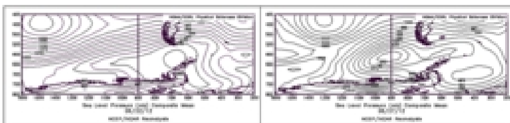
Рис. 9. Поля давления, приведенного к уровню моря, 22 и 27 июня 2012 г.
