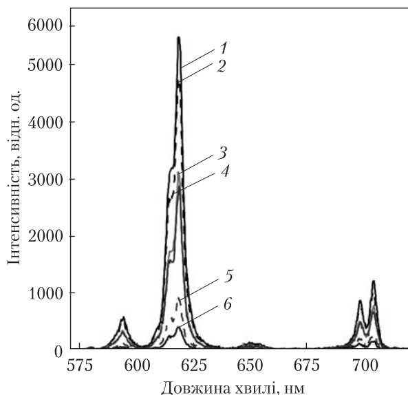
Рис. 5. Залежність люмінесценції донора (наночастинки \text{GdVO}_4:\text{Eu}^{3+} ) від концентрації метиленового синього (МС): 1 – [\text{МС}] = 0 \text{ М} ; 2 – [\text{МС}] = 1 \cdot 10^{-6} \text{ М} ; 3 – [\text{МС}] = 5 \cdot 10^{-6} \text{ М} ; 4 – [\text{МС}] = 1 \cdot 10^{-5} \text{ М} ; 5 – [\text{МС}] = 5 \cdot 10^{-5} \text{ М} ; 6 – [\text{МС}] = 1 \cdot 10^{-4} \text{ М}
