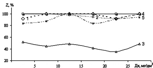
Рис.1. Влияние дозы Полвак-68 ( D_k ) на степень очистки воды от урана ( Z ) при совместном использовании с РИКС-А0 (1, 2), Al_2(SO_4)_3 (3) и FeSO_4 при разных дозах D_k , мг/дм 3 : 1, 3, 4 – 10; 2, 5 – 20.
