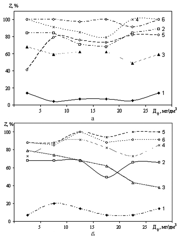
Рис.2. Влияние дозы флокулянтов ( D_f ) CWL-40 (а) и Magnafloc-351 (б) на степень очистки воды от урана (Z) при расходе коагулянтов РИКС-А0 (1–5) и Полвак-68 (6), мг/дм 3 : 1 – 0 (рН 8,0); 2 – 10 (рН 4,0); 3 – 10 (рН 6,0); 4 – 10 (рН 8,0); 5 – 20 (рН 8,0); 6 – 10 (рН 8,0).
