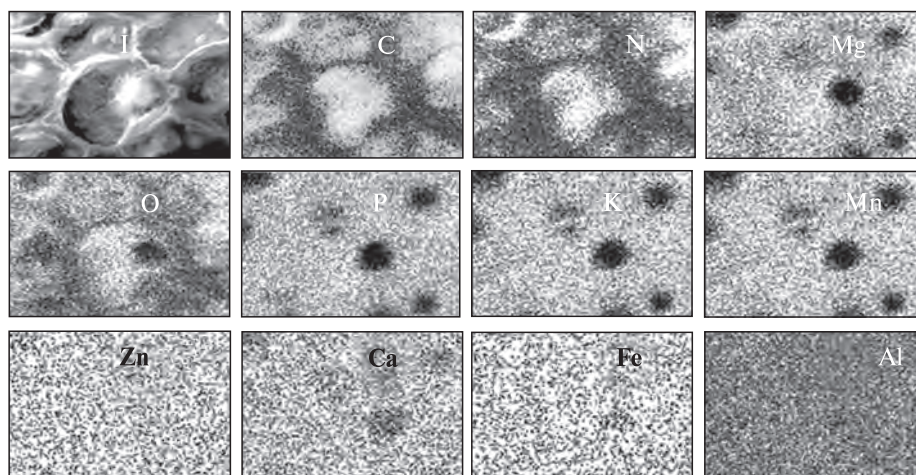
Рис. 3. Рентгенофлуоресцентные карты распределения элементов в клетках запасающей паренхимы семядолей льна сорта McGreggor: I – нативное изображение клеток в режиме низкого вакуума. Темные точки на изображениях соответствуют сигналам эмиссионных квантов элементов: С – углерода, Mg – магния, О – кислорода, Р – фосфора, К – калия, Mn – марганца, Zn – цинка, Са – кальция, Fe – железа, Al – алюминия. Высокая плотность точек на изображениях соответствует высокой концентрации элемента в компартментах клеток. Ув. 5000
