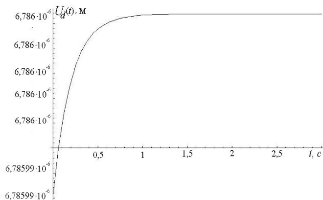
Рис. 2. Часова залежність U_d(t) = cU_0(1 - e^{-t/\tau}) , яку визначено для лишків \eta = 0 , \eta = -1/(k\tau) компоненти тензора M_{xz}
