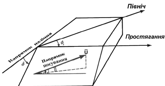
Рис. 1. Геометрія дислокаційної моделі
