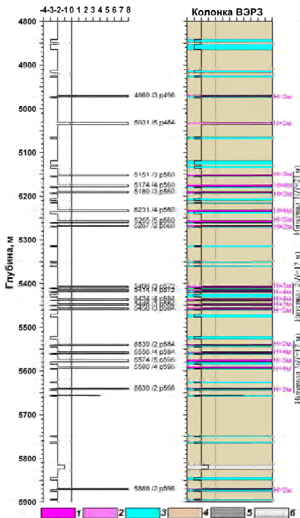
Рис. 7. Результаты зондирования ВЭРЗ в пункте VI. Аномально поляризованный пласт типа: 1 – “газ”, 2 – “газ с небольшим пластовым давлением”, 3 – “вода”, 4 – “аргиллит-алевролит”, 5 – “песчаник” (коллектор газа и воды), 6 – “известняк”; 5869/2 p596 – глубина залегания АПП типа “газ”, м, его мощность, м, значение пластового давления, атм (1 атм ≈ 0,1 МПа) соответственно
