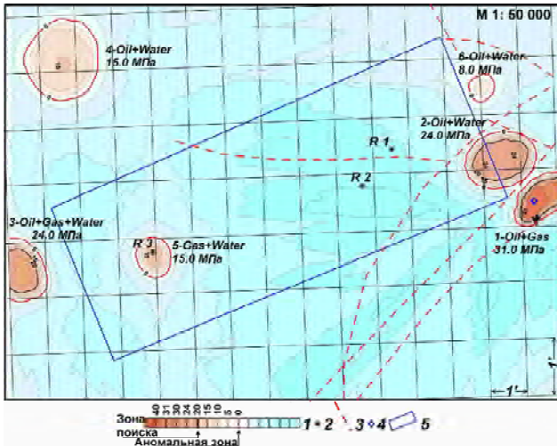
Рис. 10. Карта аномальных зон типа “залежь УВ” на участке обследования в пределах лицензионной площади Захатсор (по результатам частотно-резонансного анализа спутниковых данных), Республика Казахстан: 1 – шкала значений комплексного параметра пластового давления, МПа; 2 – положение проектных скважин; 3 – тектоническое нарушение по результатам обработки спутниковых данных; 4 – центральная часть аномальной зоны 1-Oil+Gas; 5 – контур поискового участка
