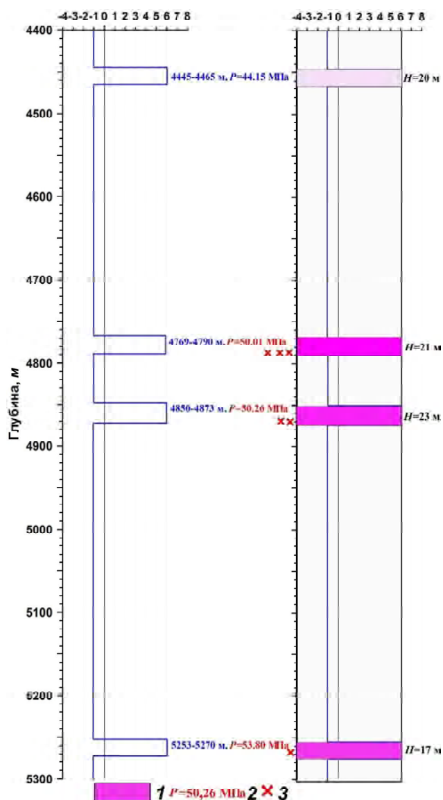
Рис. 2. Результаты вертикального частотно-резонансного сканирования данных ДЗЗ в районе поисковой скважины Беляевская-400 (Днепровско-Донецкая впадина): 1 – аномально поляризованный пласт (АПП) типа “газ”; 2 – значение комплексного параметра пластового давления в АПП; 3 – перспективные интервалы (пласты) поисков газа
