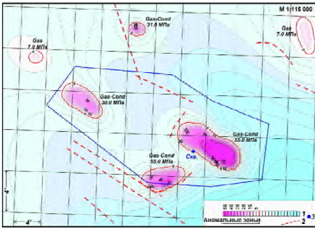
Рис. 3. Карта аномальных зон типа “газовая залежь” в районе бурения разведочной скважины Новомечевилловская-100 в Близнюковском р-не Харьковской обл. (по результатам частотно-резонансной обработки и интерпретации данных ДЗЗ): 1 – шкала максимальных значений пластового давления, МПа; 2 – тектоническое нарушение; 3 – положение скв. Новомечевилловская-100
