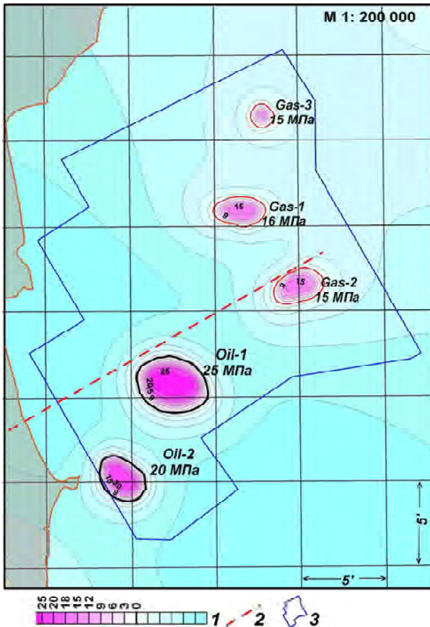
Рис. 11. Карта аномальных зон типа “нефтегазовая залежь” в районе расположения поисковой площади на шельфе Тринидад и Тобаго (по результатам обработки и дешифрирования данных ДЗЗ): 1 – шкала интенсивности аномального отклика (в максимальных значениях пластового давления, МПа); 2 – тектонические нарушения (по результатам обработки данных ДЗЗ); 3 – контур поисковой площади
