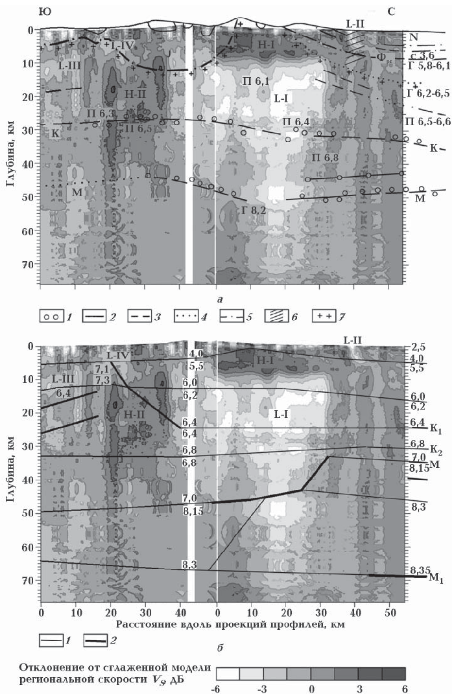
Рис. 7. Микросейсмическое зондирование по профилю Цхинвали—Ардон и результаты интерпретация центральной части профиля ГСЗ Бакуриани—Степное в интерпретации Г. В. Краснопецовой и Г. А. Павленковой: а — сейсмогеологический разрез в интерпретации [Краснопецова и др., 1970] (1 — значения глубин отражающих горизонтов с разных пунктов взрыва; 2, 3 — участки границ, построенные по уверенным сейсмическим данным (2), по менее уверенным (3); 4 — участки интерполяции границ; 5 — границы, построенные по геологическим данным; б — зоны нарушения корреляции сейсмических волн; 7 — поверхность «гранитного» слоя по сейсмическим данным). Скорости сейсмических волн, км/с: г — граничная, п — пластовая, с — средняя для осадочной (мезозойско-кайнозойской) толщи Предкавказского прогиба. Ф пз — поверхность палеозойского фундамента; К — граница, связанная с «базальтовым» слоем или его аналогами; М — граница Мохоровичича; N, J — обобщенный возраст слоев отложений (неоген-четвертичный и юрский соответственно); б — скоростной разрез в интерпретации [Павленкова, 2012] (1 — границы между слоями с разными сейсмическими скоростями; 2 — отражающие площадки; K1 и K2 — внутрикоровые границы; M — граница Мохоровичича, M1 — внутримантийная граница. Ссылки на зоны с индексами Н и Л см. в тексте.
