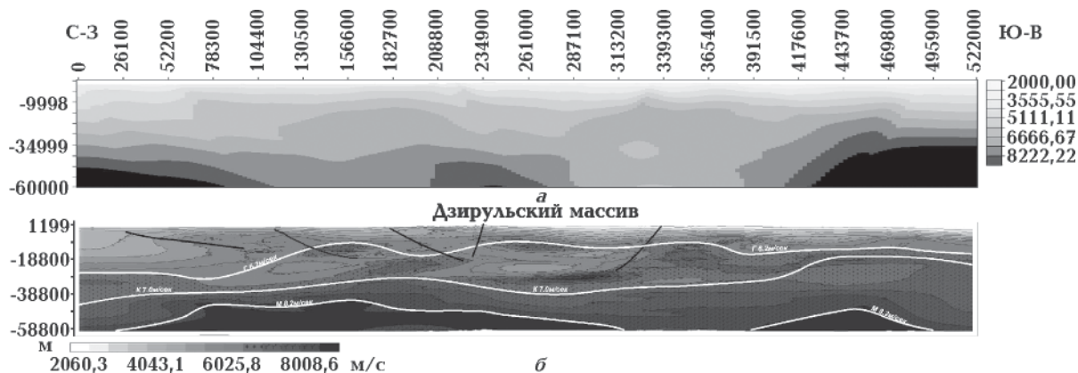
Рис. 5. Сейсмотомография ГСЗ профиля Гали—Сафаралиев: а — томография XТото-LM2, б — томография GeoGiga.
