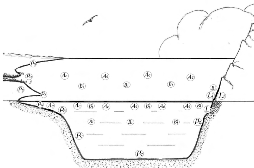
7. Распределение контурных биотопов и их сообществ в морской среде (схема): Ac — аэроконтур; Ps — псаммоконтур; Li — литоконтур; Pe — пелоконтур; Po — потамоконтур; Bi — биоконтур.
