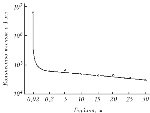
2. Среднегодовая численность бактерий (кл·см -3 ) на разных горизонтах водной толщи в северо-западной части Черного моря [47].
