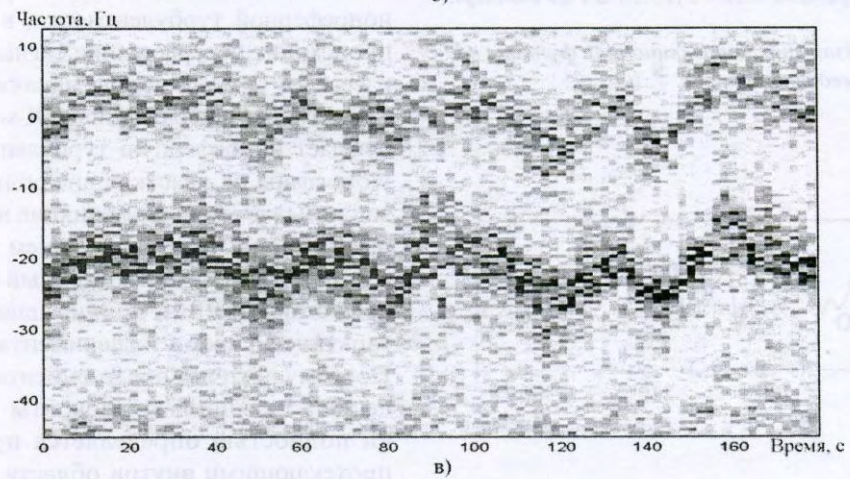
Рис. 6. Спектрограммы сигнала НС, принятого в 4:34–4:37 UT, 29.10.2002 г.: а) в Антарктике на УАС “Академик Вернадский”, б) в РАО РИ НАНУ, в) вблизи Санкт-Петербурга
