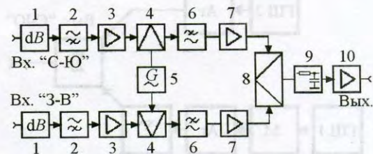
Рис. 1. Функциональная схема двухканального широкополосного корреляционного приёмника: 1 – аттенюатор (0 ÷ 31 дБ), 2 – фильтр ВЧ ( f_{cp} = 18 МГц), 3 – усилитель ВЧ ( K = 6 дБ), 4 – балансный смеситель, 5 – гетеродин (Г4-1А), 6 – фильтр НЧ ( f_{cp} = 0.5 МГц), 7 – видеоусилитель ( K = 90 дБ), 8 – перемножитель, 9 – интегратор ( \tau = 10^{-1}, 10^{-2} с), 10 – усилитель постоянного тока
