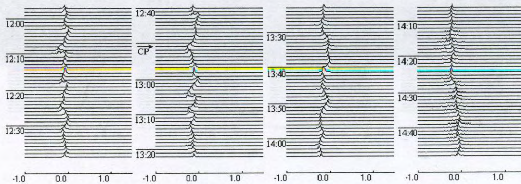
Рис. 6. Вариации ДС на частоте 3.5 МГц при старте ракеты "Delta" в 12:51 7 октября 1999 г. (действующая высота 315 \pm 390 км)
