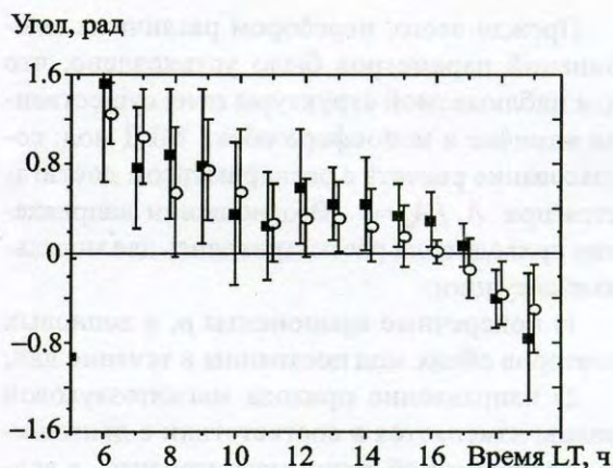
Рис. 6. Позиционный угол эллипса поляризации геомагнитных пульсаций. Сравнение результатов эксперимента (22.03 – 31.03.1998 г. “Академик Вернадский”) и моделирования: ■ – экспериментальные данные, ○ – результат моделирования
