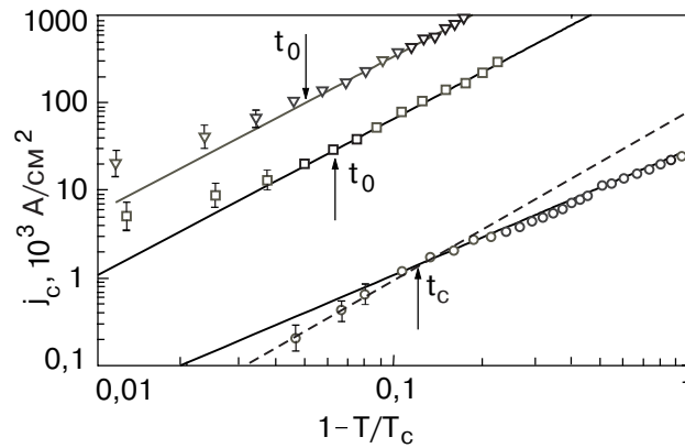
Рис. 3. Температурные зависимости плотности критических токов образцов W62 (○), W136 (□) и W154 (▽) в двойных логарифмических координатах; прямые — уравнения j_c(T) = j_c(0)(1 - T/T_c)^s , построенные для каждого образца с теми же значениями параметров j_c(0) и s , что на рис. 2; пунктир — зависимость j_c(T) \sim t^2 . Стрелками обозначены температуры t_0 для образцов W154 и W136 и t_c для образца W62.
