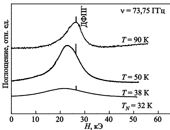
Рис. 8. Спектры ЭПР кристалла \text{Nd}_{0,75}\text{Dy}_{0,25}\text{Fe}_3(\text{BO}_3)_4 при температурах 38, 50 и 90 К при \mathbf{H} \parallel \mathbf{c} .
