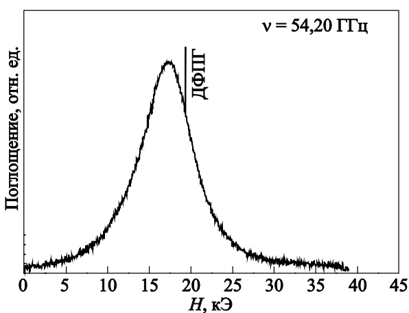
Рис. 9. Спектр ЭПР кристалла \text{Nd}_{0,75}\text{Dy}_{0,25}\text{Fe}_3(\text{BO}_3)_4 при T = 50 К и \mathbf{H} \perp \mathbf{c} .
