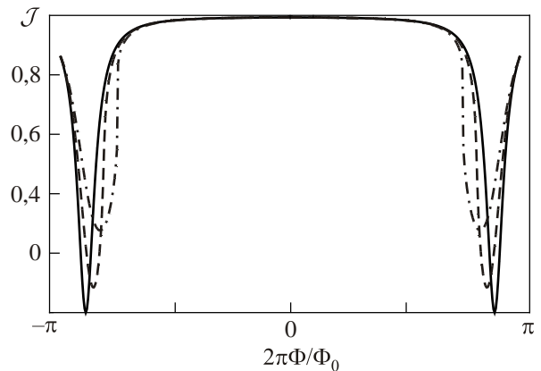
Рис. 5. Зависимость коэффициента прохождения от значения потока через петлю. Вычисления проведены для случая идентичных джозефсоновских переходов, I_{C1} = I_{C2} = 5 \cdot 10^{-7} А, C = 10^{-12} Ф, R = 10^4 Ом, Z_l = 57 Ом, \omega_J = 5,5 \cdot 10^{10} с ^{-1} , \omega = 0,6 \omega_J , I_0/I_{C1} = 0,25 — пунктирная линия, I_0/I_{C1} = 0,4 — штрихпунктирная линия. Сплошная линия соответствует линейному приближению и построена для указанных параметров согласно (24).
