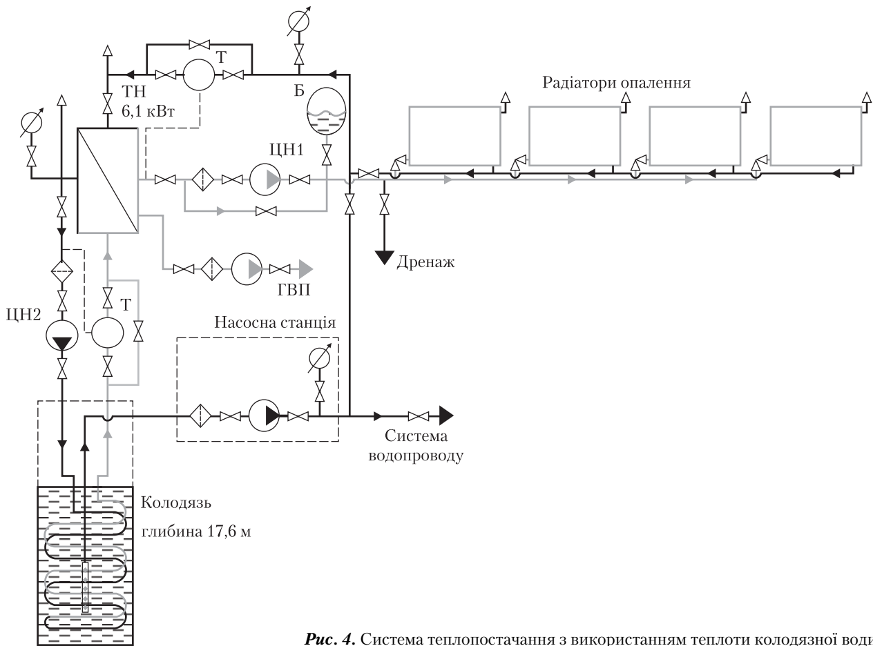
Рис. 4. Система теплопостачання з використанням теплоти колодезяної води
