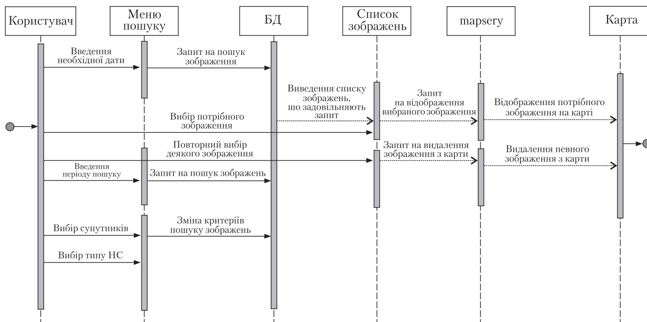
Рис. 9. Діаграма послідовностей використання системи
