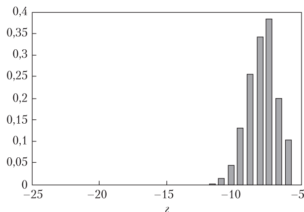
Рис. 3. Гістограма значень коефіцієнта зворотного розсіювання ( \gamma dB) на радіолокаційному зображенні Envisat/ASAR для: a – підтопленої рослинності; б – відкритої води; в – пісків та відкритих ґрунтів; г – рослинності
