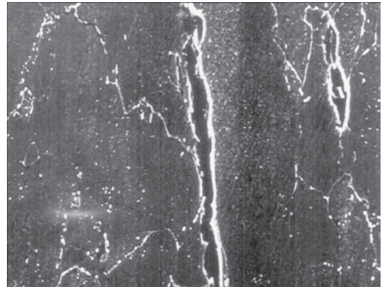
Рис. 9. Трещина ползучести в сварном соединении. Нароботка 280000 ч ( \times 2500 )
