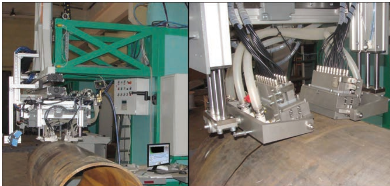
Установка НК 362MB для АУЗК концевых участков труб большого диаметра, поставлена на ОАО «Выксунский металлургический завод», 2013 г.
