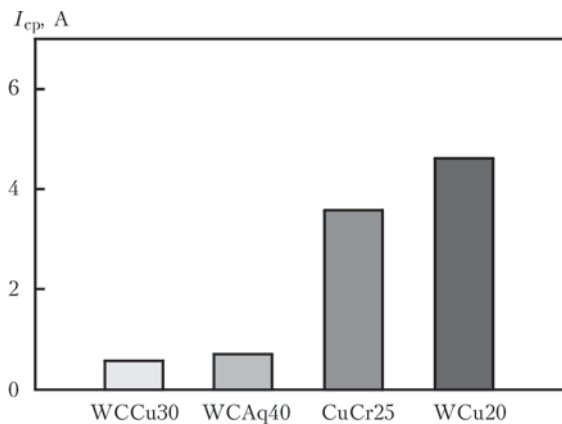
Рис. 3. Ток среза для различных контактных материалов при испытаниях вакуумного контактора 24 кА/24 кВ при максимальном токе 30 А [26]
