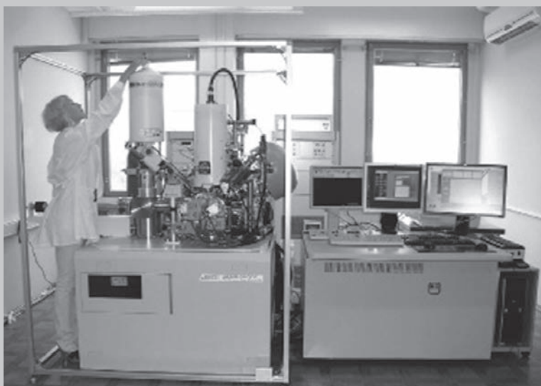
Оже-микросонд с полевым эмиссионным катодом JAMP-9500F (JEOL Ltd, Япония), укомплектованный энергодисперсионным спектрометром OXFORD EDS INCA Energy 350 для анализа элементов от бериллия до урана.
