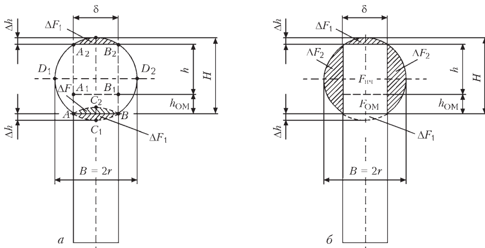
Рис. 3. Основные показатели поперечного сечения валика при однослойной наплавке на узкую подложку (обозначения см. в табл. 1). Заштрихованные части валика (б) удаляются при механической обработке наплавленного металла
