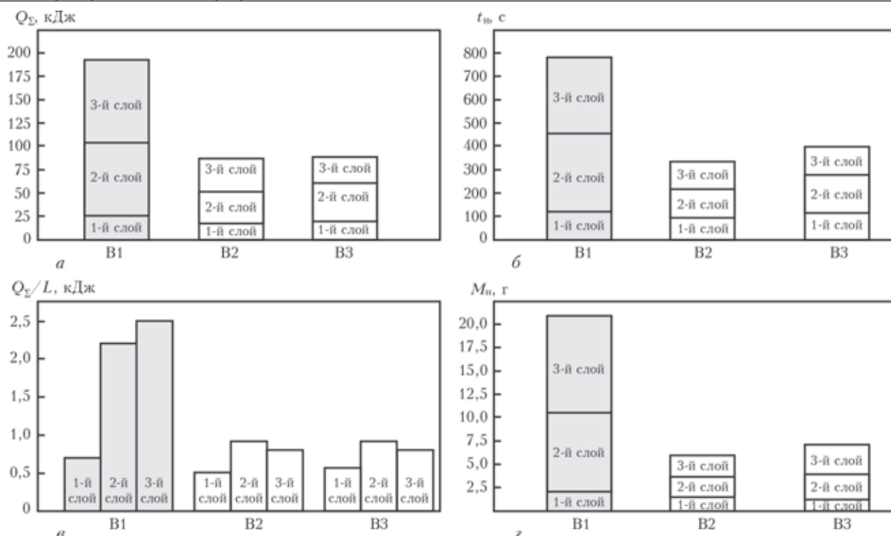
Рис. 8. Закономерности изменения количества тепла Q_{\Sigma} , вводимого в изделие, времени наплавки t_{н} и средней величины сварочного тока I при коррекции режимов наплавки узкой подложки переменной ширины \delta = 2,5 \dots 6,0 мм: B1 — установка УПНС-304M2/M3, защитный газ Ar + 10\% H_2 ; B2 — установка УПНС-304M2/M3, защитный газ Ar + 5\% H_2 ; B3 — установка STARWELD PTA 190H фирмы «Kennametal Stellite GmbH», защитный газ Ar . Присадочный порошок — сплав ЖС32. Темным цветом выделен режим наплавки, где проявляется склонность к образованию микротрещин
