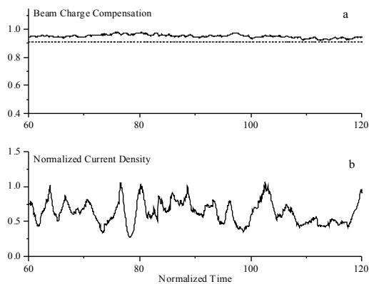
Рис. 6. Степень зарядовой компенсации (а) и плотность пучка (б) в режиме статистического равновесия. Пунктиром отмечено критическое значение степени компенсации
