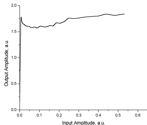
Рис. 7. Зависимость амплитуды выходного сигнала от амплитуды входного сигнала в ЛБВ усилителе с ионной фокусировкой электронного пучка
