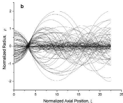
Рис. 2. Перемешивание фаз бетатронных колебаний и образование равновесного пучка
