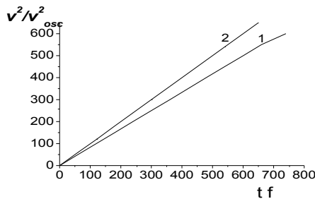
Рис.3. Зависимость отношения квадратов скоростей электрона V^2/V_{osc}^2 от безразмерного времени t*f . Кривая 1 – рост отношения V^2/V_{osc}^2 от t*f при движении электрона в поле МВИССФ; кривая 2 – рост отношения V^2/V_{osc}^2 от t*f при движении электрона в поле с регулярными скачками фазы на \pi через n периодов поля волны [9]
