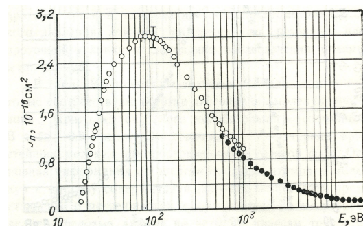
Рис.1. Зависимость сечения ионизации от энергии электрона для аргона
