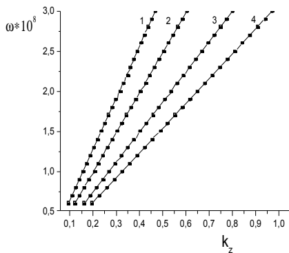
Рис.2. Зависимость частоты \omega от продольного волнового числа k_z \equiv k_z для четырех радиальных веток плазменных волн: четвертой радиальной (кривая 4), третьей радиальной (кривая 3), второй радиальной (кривая 2), первой радиальной (кривая 1) (при изменении частоты в диапазоне от \omega=6 \cdot 10^8 \text{ с}^{-1} до \omega=3 \cdot 10^9 \text{ с}^{-1} для приведенных выше параметров плазмы и волновода)
