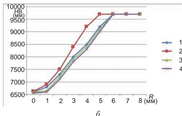
Рис. 2. Графики изменения твердости шаров различных размеров: а — по поверхности шара, б — вглубь шара
