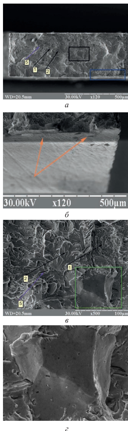
Рис. 7. Разрыв на участках образцов третьего типа: а — общий вид с отмеченными особенностями, б — увеличение изображения участка с сужением шейки (длинная прямоугольная рамка на рис. 7а), в — увеличение изображения участка образца (прямоугольная рамка на рис. 7а, черная), г — область с полостями (прямоугольная рамка на рис. 7в)
